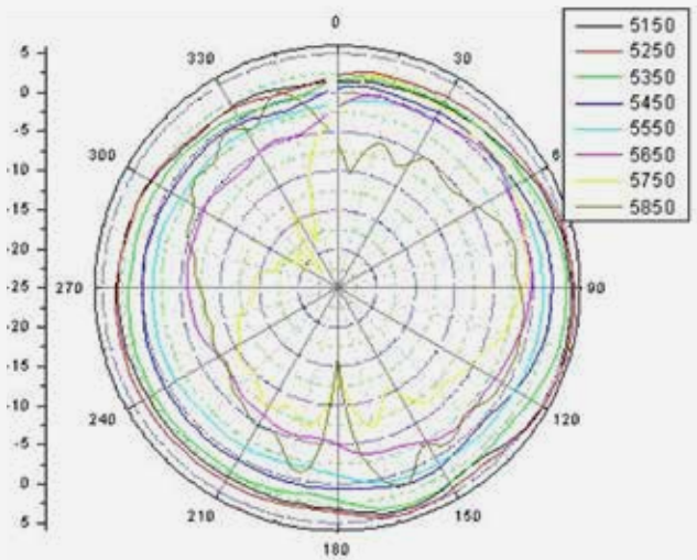
5G (PHI=90)
