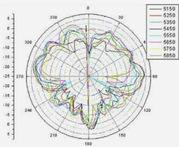
5G (PHI=0)
