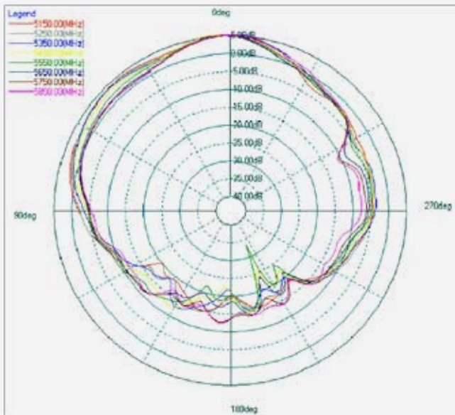
5G (PHI=0)
