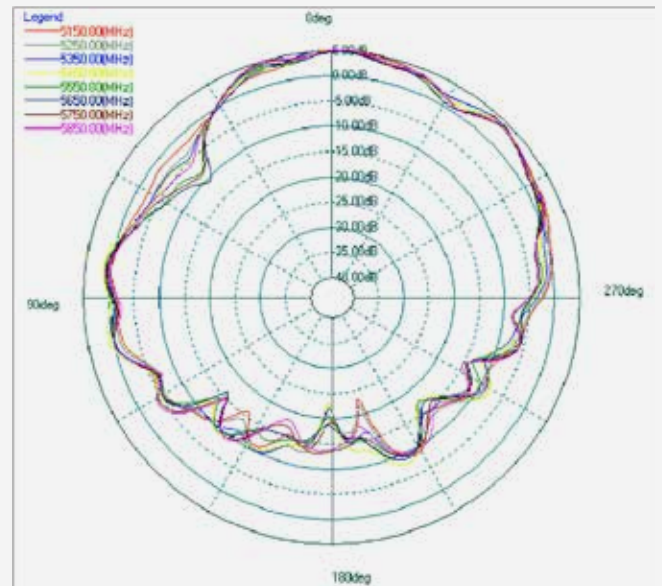
5G (PHI=90)
